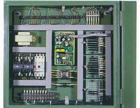
電控箱元件，控制動作以無接點開關控制幾乎無壽命問題
